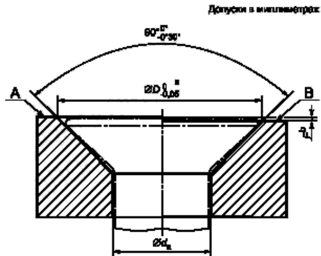
Рисунок 2 — Потайной калибр
